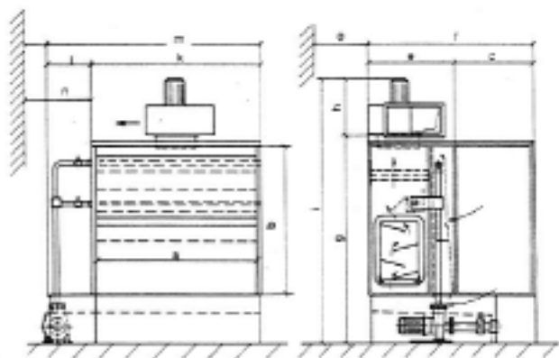
Wasserbeflutete-Spritzkabine Typ: SKW
